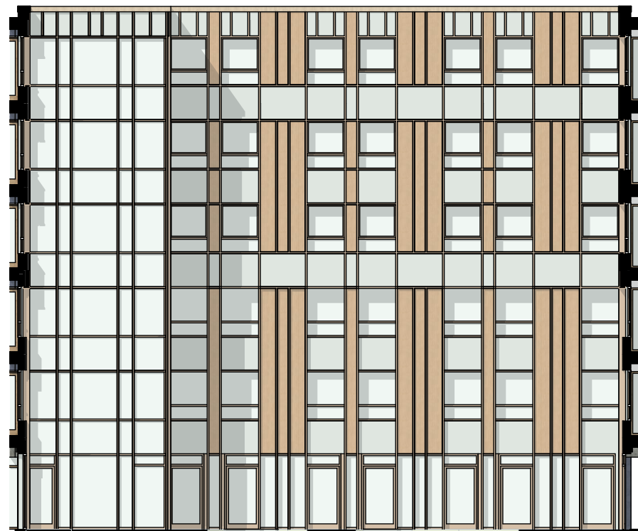
noordgevel
